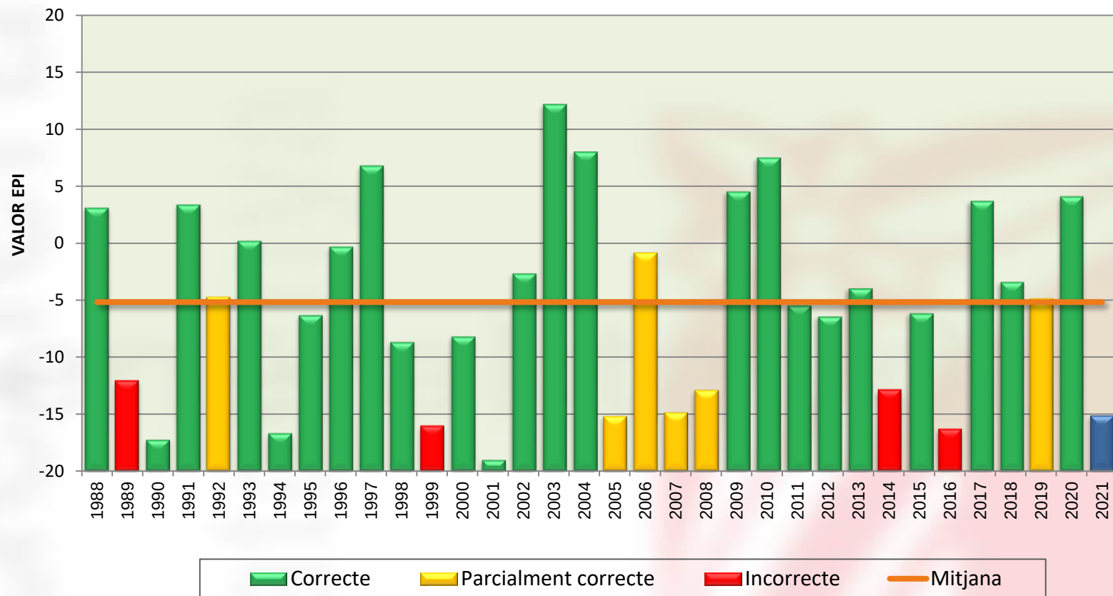
Valor EPI hivernal Vilafranca del Penedès (1988-2021)
